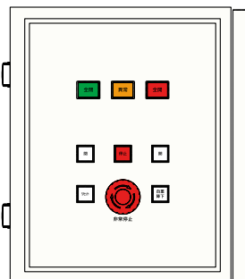
別置操作盤
